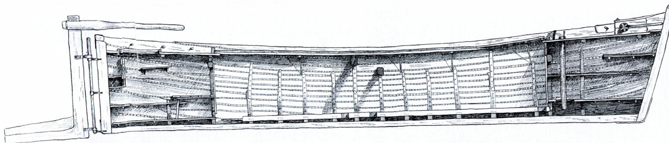
Peipsi lodja pikiläbilõige
